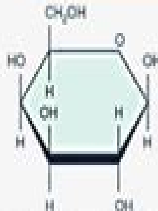
GALACTOSE
