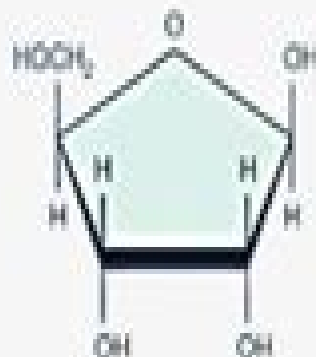
RIBOSE
