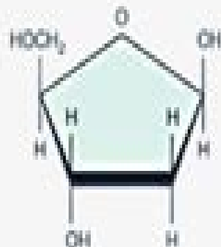
DEOXYRIBOSE
