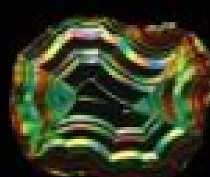
Iris Agate
