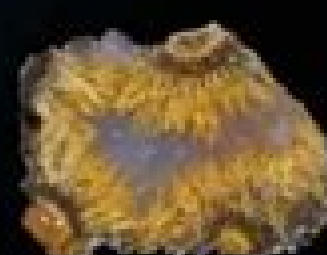
Sagenite Agate
