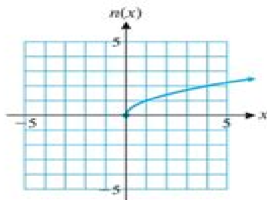
(D) Square root function
