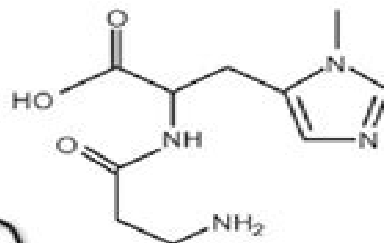
Anserine
