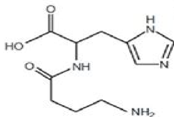
Homocarnosine
