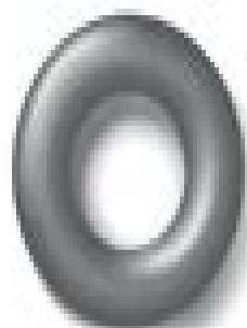
TORUS
