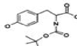
N-t-Boc Tyrosine
